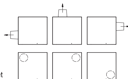
Mögliche Einbauvarianten Ø 75/80 hinten: (von vorne gesehen)
