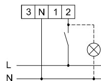
Schaltbild 1: einstufige Ausführung Ein/Aus über baueifügen Schalter
